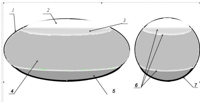
Şəkil 1. Kainatdakı Müqəddəs İşıq çalarlarının paylanması sxemi
