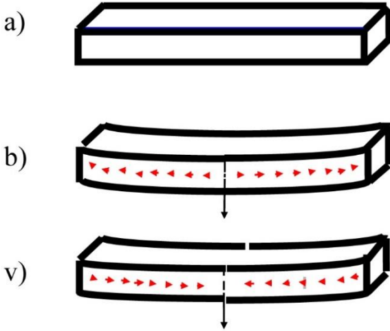
Şəkil 5. Zəlzələ anında yer laylarında dartılma və çökmə sxemi
