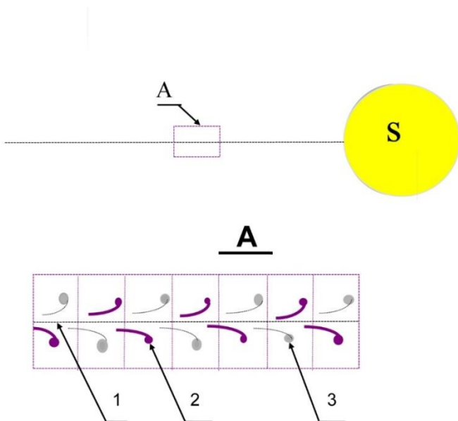
Şəkil 3. Günəş İşığı zərrəsinin formalaşması sxemi.
