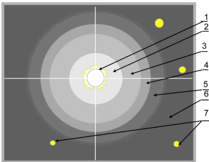
Şəkil 4. Günəş haləsinin rəngləri (miqyas gözlənilməmişdir)
