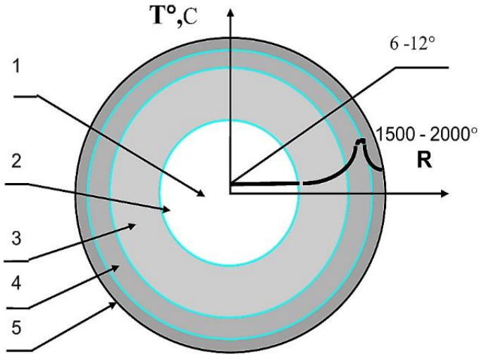
Şəkil 2. Günəş cisminin kəsiyinin sxematik quruluşu
