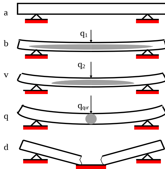
Tirin yüklənmə sxemi
