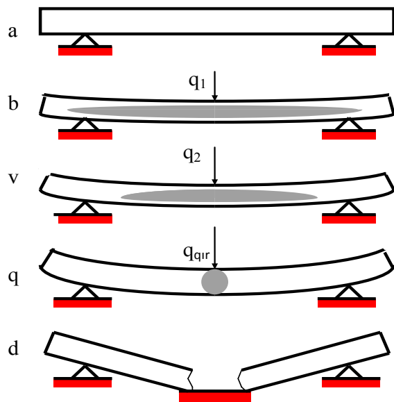
Tirin yüklənmə sxemi
