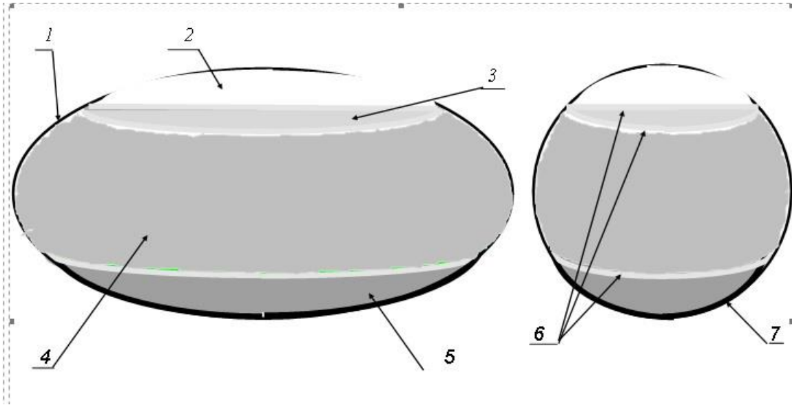
Şəkil 1. Kainatdakı Müqəddəs Işıq çalarlarının paylanması sxemi
