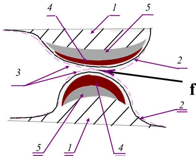
Şəkil 9. Cisimlərin səthlərindəki çıxıntıların ətrafında zərrələrin paylanma sxemi
