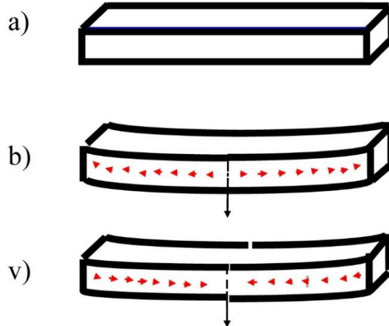
Şəkil 5. Zəlzələ anında yer laylarında dartılma və çökmə sxemi
