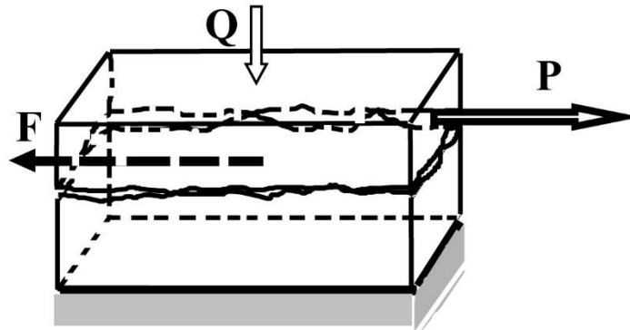
Şəkil 8. İki sürtünən cismə tə'sir edən qüvvələr sistemi
