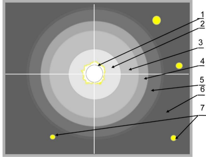
Şəkil 4. Günəş haləsinin rəngləri (miqyas gözlənilməmişdir)
