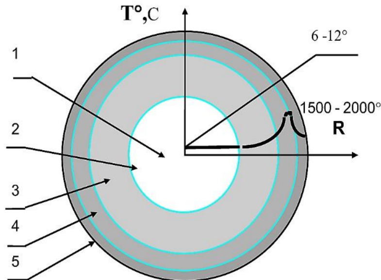
Şəkil 2. Günəş cisminin kəsiyinin sxematik quruluşu
