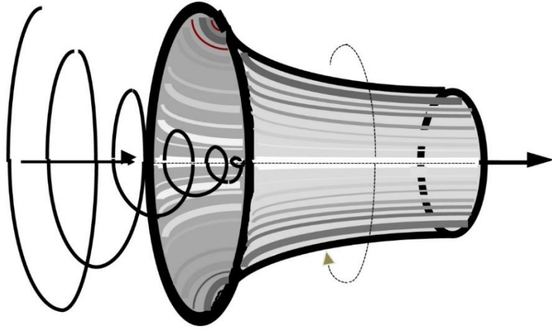
Şəkil 7. Kainatda qara çuxurun — burulğanın quruluşu və sxematik iş prinsipi
