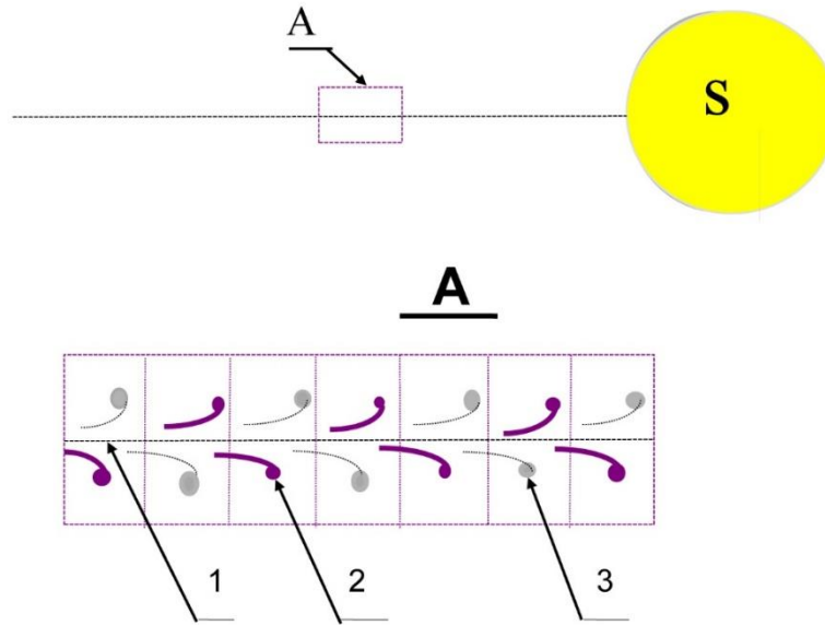
Şəkil 3. Günəş işığı zərrəsinin formalaşması sxemi.
