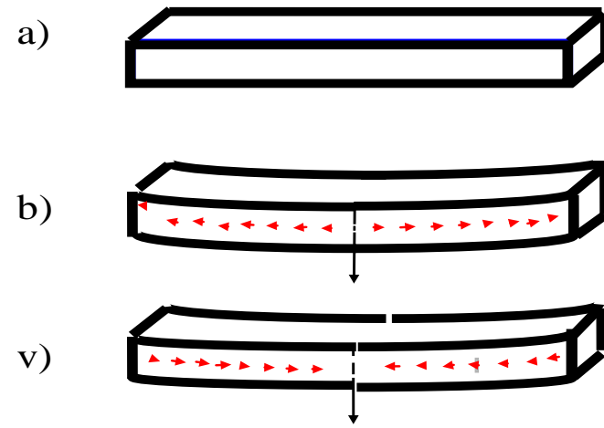
Şəkil 5. Zəlzələ anında yer laylarında dartılma və çökmə sxemi
